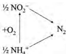
Рис. 2. Схема анамокс-процесу
