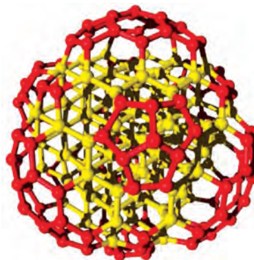
Рис. 3. Кристалічна структура нанодіамантів: можлива структура вуглецевого кластера C_{275} , який має ядро діаманта sp^3 1,4 нм у діаметрі (жовтий колір) та фулереноподібну відновлену поверхню sp^2 (червоний колір) [53]
