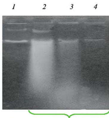
Рис. 5. Електрофореграма ДНК плазмиди pGLG578, розщепленої ДНКазою I: 1 — нативна ДНК; 2 — ДНК після оброблення ДНКазою I у концентрації 0,05 U/мкг ДНК; 3 — ДНК після оброблення ДНКазою I у концентрації 0,1 U/мкг ДНК; 4 — ДНК після оброблення ДНКазою I у концентрації 0,5 U/мкг ДНК; доріжки із розщепленою ДНК
