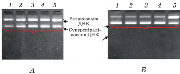
Рис. 3. Електрофореграма зразків ДНК плазмиди pGLG578 за присутності поліамфолітних носіїв БГ-3 (А) і БГ-4 (Б): до 1 мкг плазмідної ДНК додавали 1 мкл полімеру відповідної концентрації в об'ємі 9 мкл трис-НСl, 20 мМ, рН 7,4. Доріжка 1 — 0,1% полімеру, 2 — 0,03%, 3 — 0,01%, 4 — 0,003%, 5 — вільна плазмідна ДНК; — ДНК, що не зв'язалася з носієм
