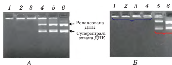
Рис. 2. Електрофореграма зразків ДНК плазмиди rGLG578 та її комплексів із поліамфолітними носіями БГ-2 (А) і БГ-2q (Б): до 1 мкг плазмідної ДНК додавали 1 мкл полімеру відповідної концентрації в об'ємі 9 мкл трис-НСl, 20 мМ, рН 7,4. Доріжка 1 — 0,1% полімеру, 2 — 0,03%, 3 — 0,01%, 4 — 0,003%, 5 — 0,001%, 6 — вільна плазмідна ДНК; — комплекс поліамфолітний носій/ДНК; — ДНК, що не зв'язалася з полімером
