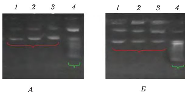
Рис. 6. Електрофоретична оцінка ДНК-протекторної здатності поліамфолітних носіїв BG-2 (А) і BG-2q (Б): до 1 мкг плазмідної ДНК pGLG578 додавали 1 мкл 0,1% -го розчину ПН в об'ємі 9 мкл трис-НСl, 20 мМ. Утворений комплекс піддавали впливу ДНКазу I у різних концентраціях: доріжка 1 — нативна ДНК; 2 — комплекс ПН/ДНК, оброблений ДНКазою I в концентрації 0,05 U/мкг ДНК; 3 — комплекс ПН/ДНК, оброблений ДНКазою I в концентрації 0,1 U/мкг ДНК; 4 — комплекс ПН/ДНК, оброблений ДНКазою I в концентрації 0,5 U/мкг ДНК; плазмідна ДНК, вивільнена з комплексу ПН/ДНК; розщеплена плазмідна ДНК
