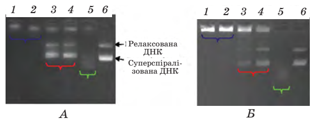
Рис. 4. Електрофореграма ДНК плазмиди pGLG578, вивільненої з комплексу з БГ-2 (А) і БГ-2q (Б):
