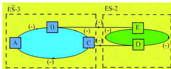
Рис. 6. Структура п'ятикомпонентного нестаціонарного епігена. Елементарні епігени: ES-3 [E-3] — осцилятор, нестаціонарний трикомпонентний епіген; ES-2 — двопозиційний модуль пам'яті, стаціонарний двокомпонентний епіген. Мінусами позначено негативні зв'язки (за [4])
