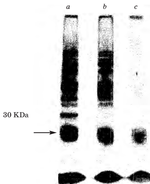
Рис. 2. Флюорографический анализ электрофоретического «спектра» полипептидов, синтезированных с помощью поли(A) ^+ РНК в бесклеточной системе из проростков пшеницы:
