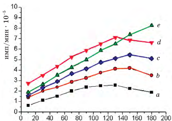
Рис. 1. Кинетика включения [^{35}\text{S}] -метионина в ТХУ-нерастворимый материал в бесклеточной системе из проростков пшеницы с использованием в качестве матрицы поли(A) ^+ РНК:
