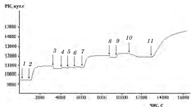
Рис. 4. Відгук ППР імуносенсора на внесення біологічних та хімічних компонентів:
